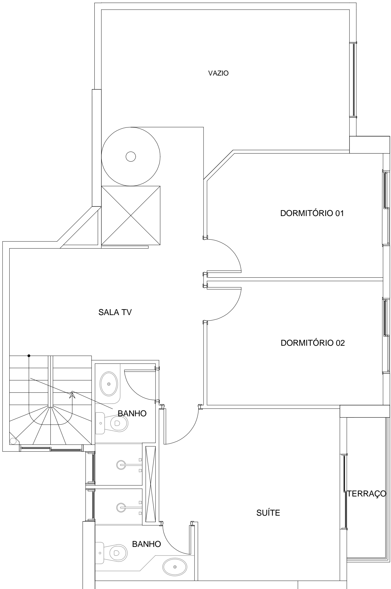
PLANTA PAVIMENTO INTERMEDIÁRIO
